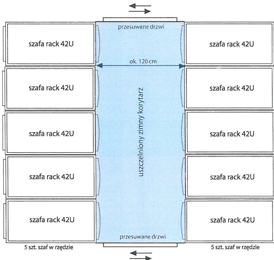
Poglądowy schemat zestawu szaf rack wraz z zabudową zimnego korytarza
